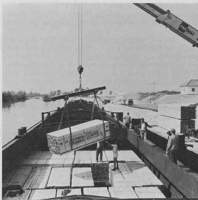
Industriehafenprojekt Enns-Ennsdorf, fertige Lände
