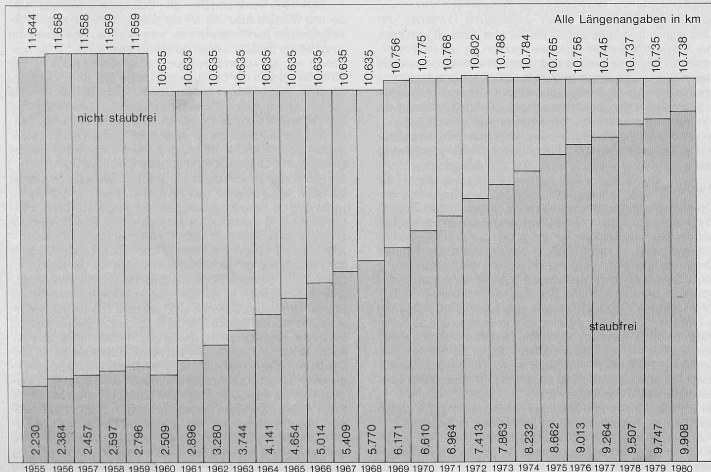
Entwicklung des Ausbauzustandes der Landeshaupt- und Landesstraßen
